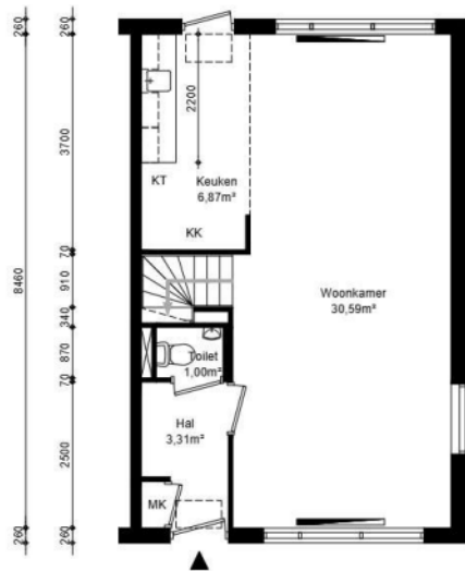
Begane grond
