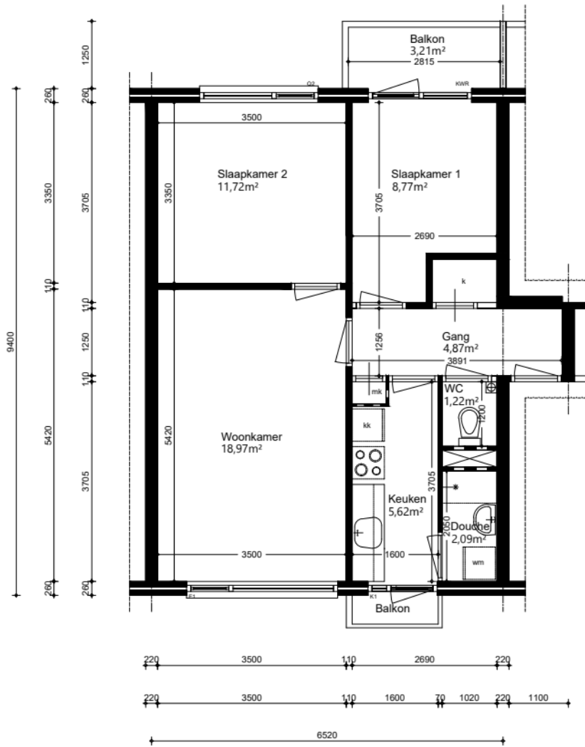
Plattegrond [woonlagen]
