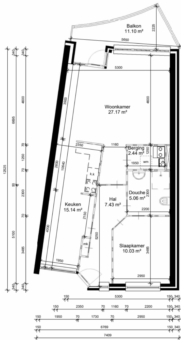
1e verdieping
