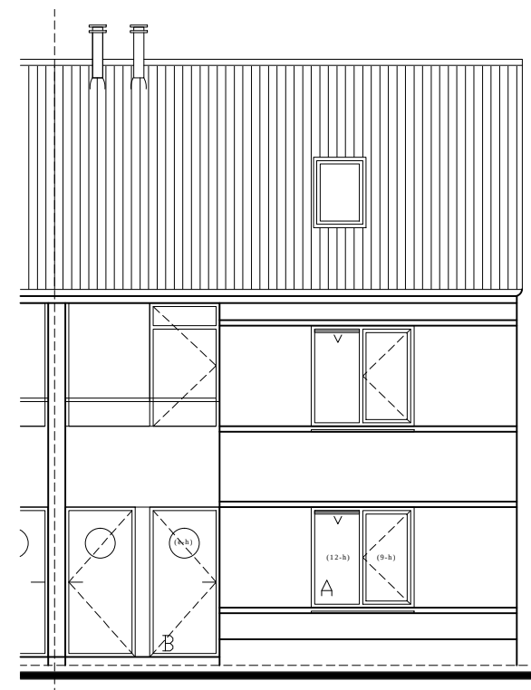
VOORGEVEL
