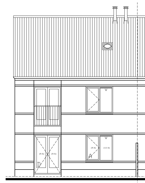
ACHTERGEVEL
