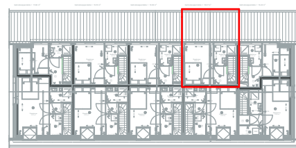
1e verdieping
