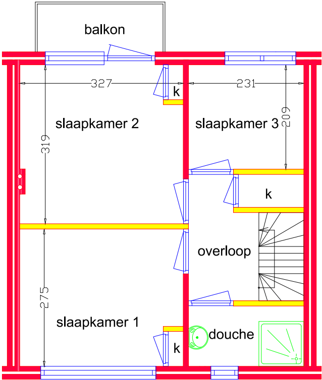
verdieping
