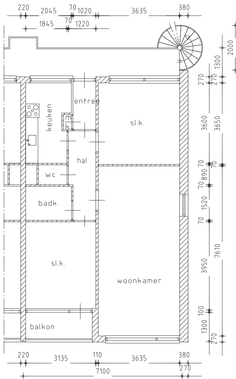
plattegrond
