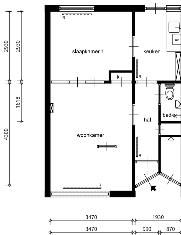
begane grond
