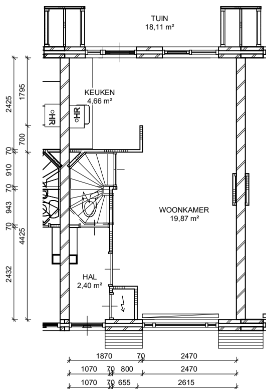
Begane grond
