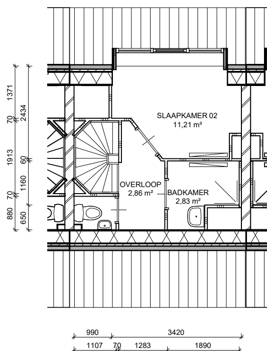
1e verdieping
