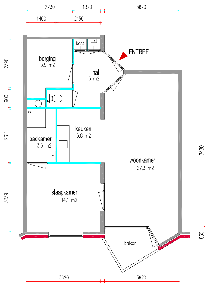
2e VERDIEPING
