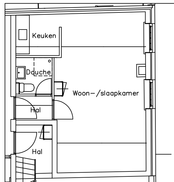
Plattegrond
