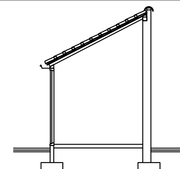
Doorsnede
