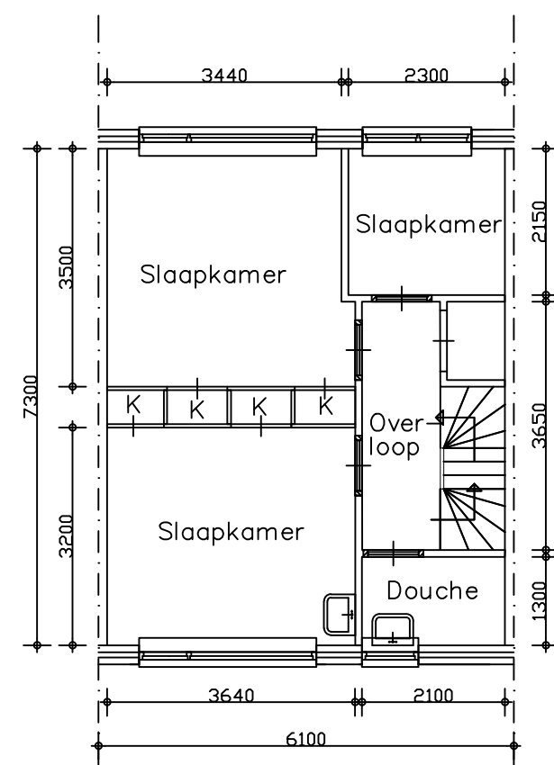
Verdieping
