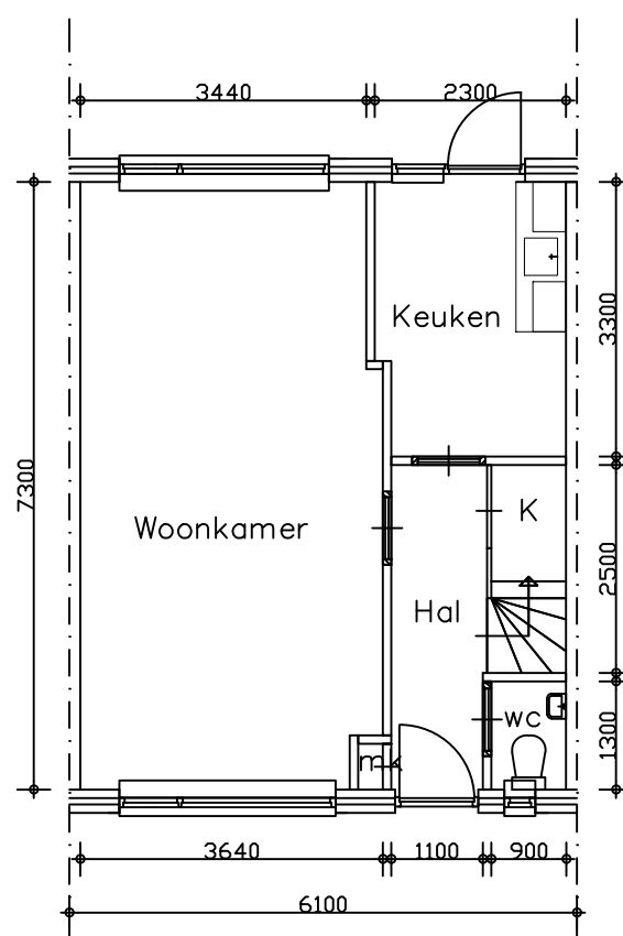
Beganegrond
