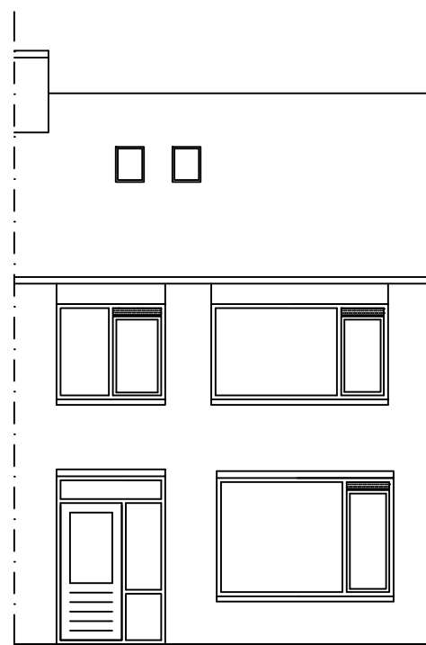
Achtergevel
