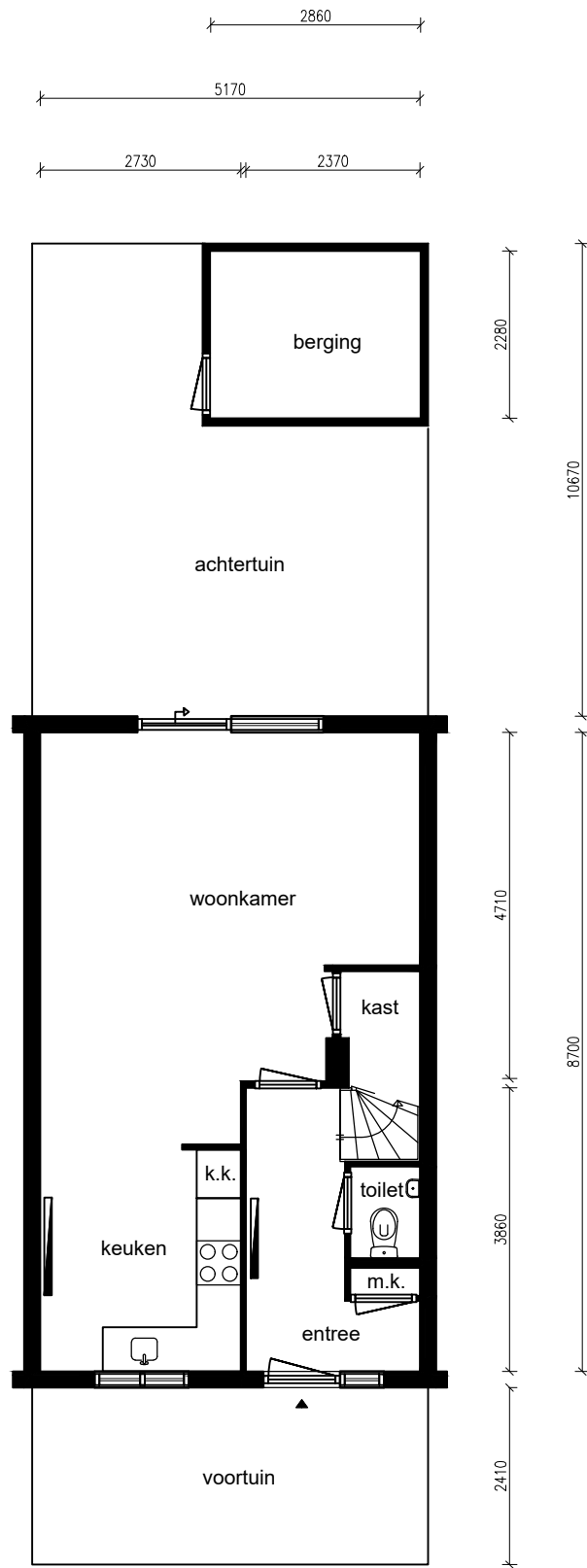
Begane grond
