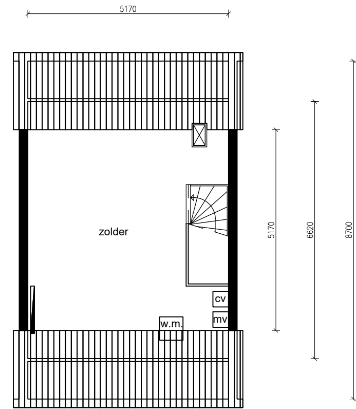
2e verdieping
