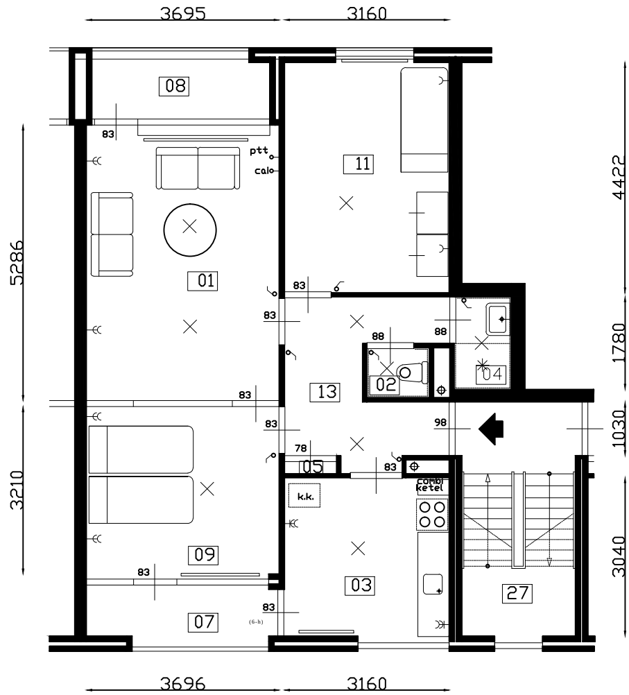
PLATTEGROND
