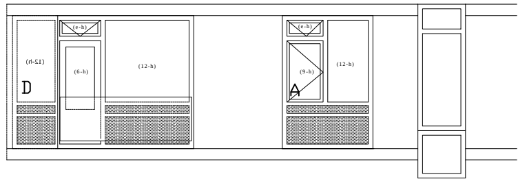
LINKERZIJGEVEL
