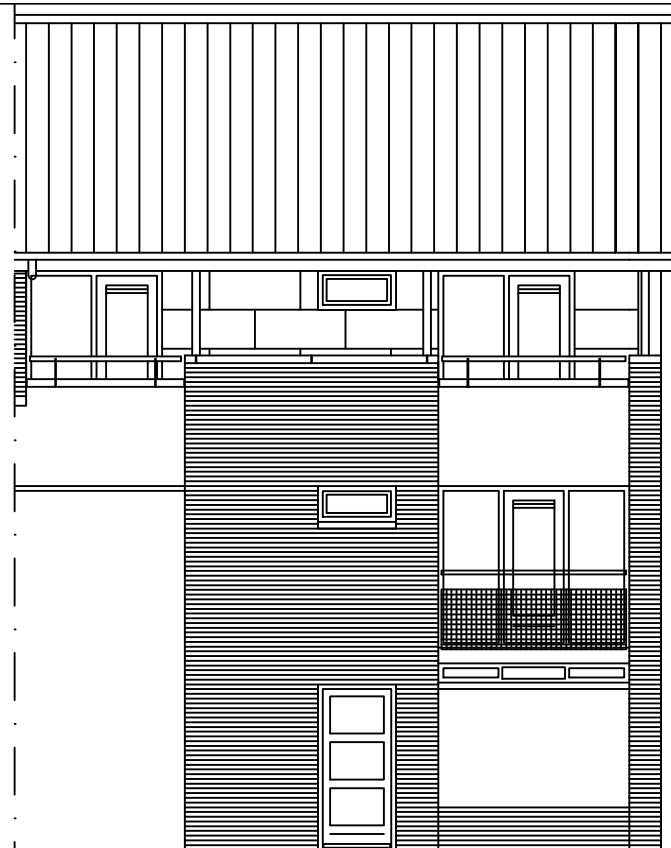
Voorgevel
