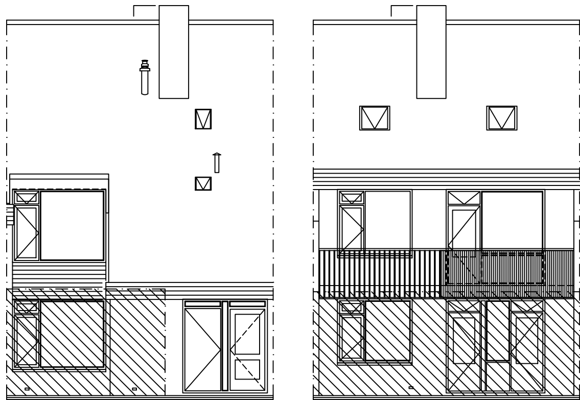
Voorgevel
