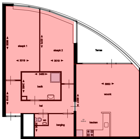
Verdieping_8e
