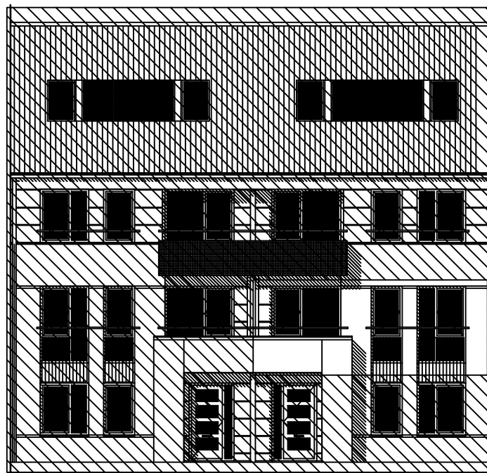
Voorgevel
