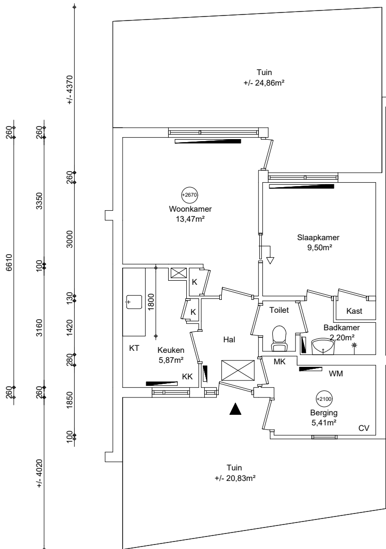
Begane grond GO wonen 43,34m 2
