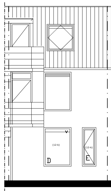
ACHTERGEVEL
