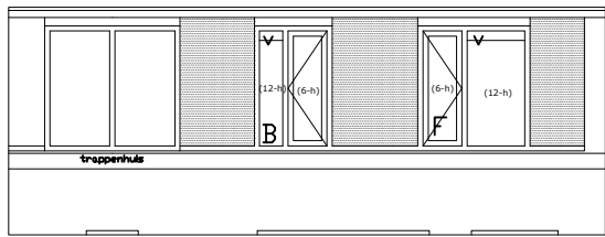
VOORGEVEL
