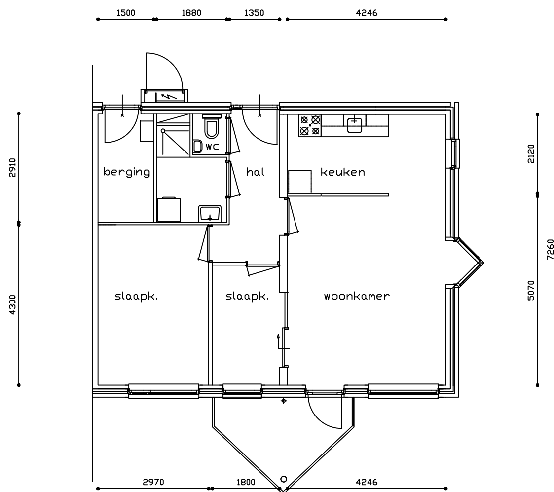
Plattegrond
