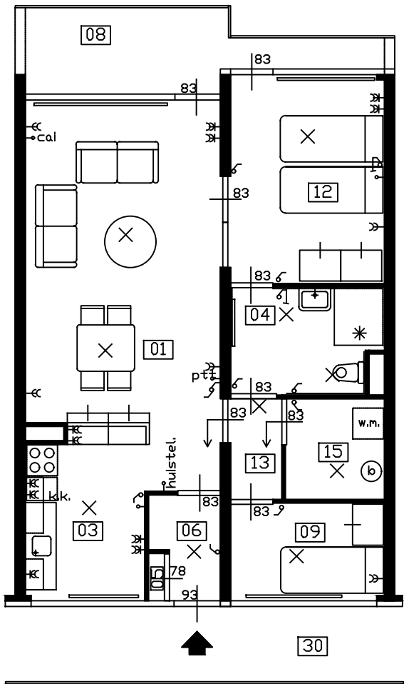
PLATTEGROND
