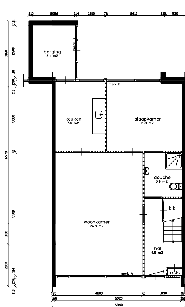
Begane grond
