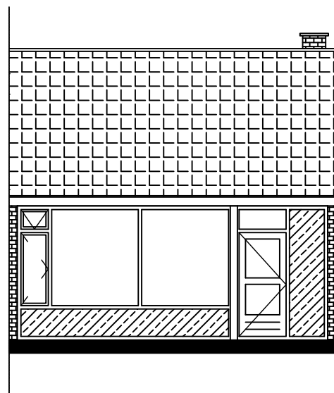
Voorgevel
