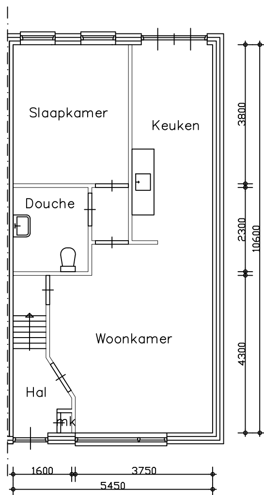
Begane grond
