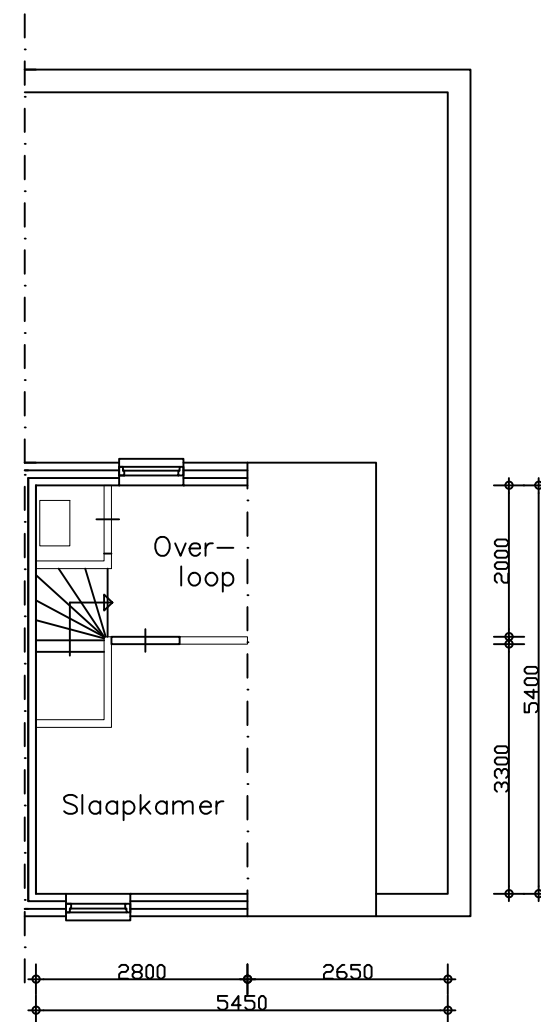
Verdieping
