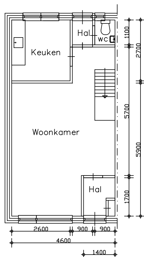
Beganegrond
