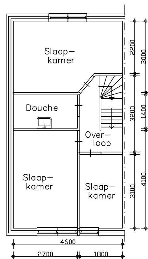
Verdieping
