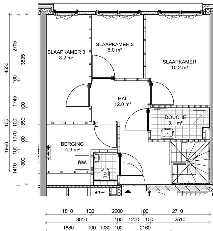
1e Verdieping
