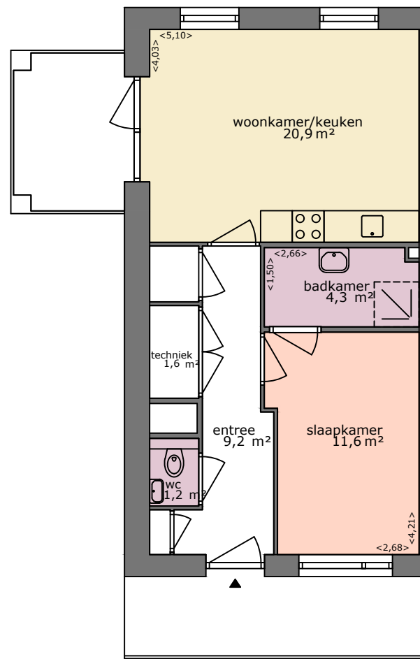
begane grond
