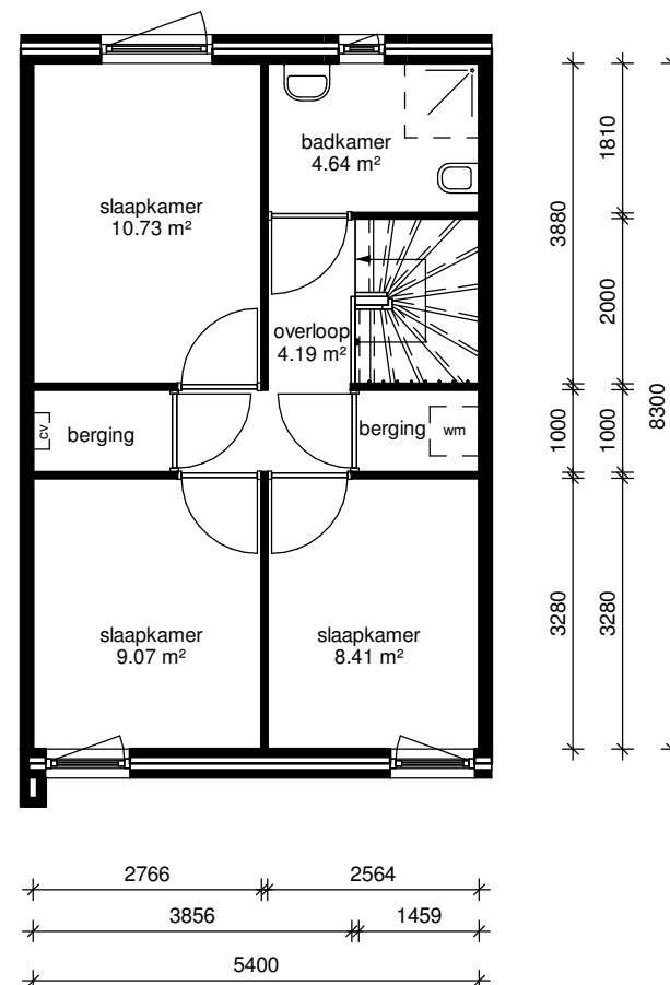
eerste verdieping
