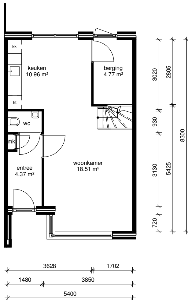
begane grond
