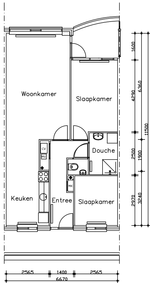
Plattegrond
