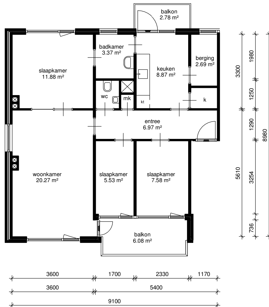
tweede verdieping
