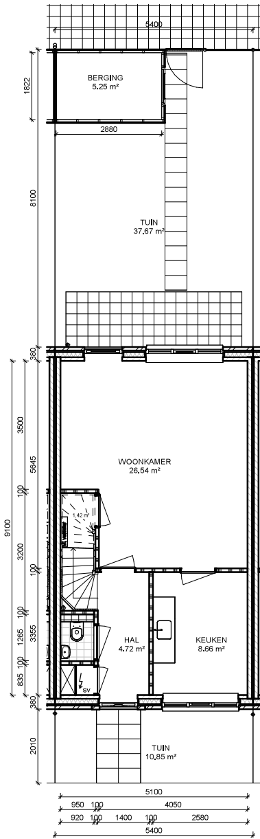
Begane grond
