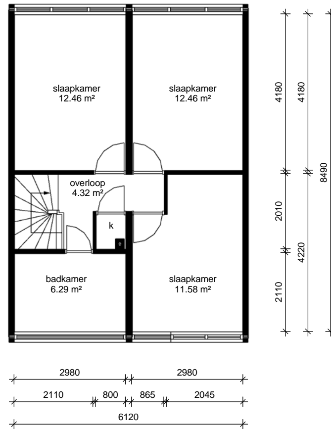
eerste verdieping
