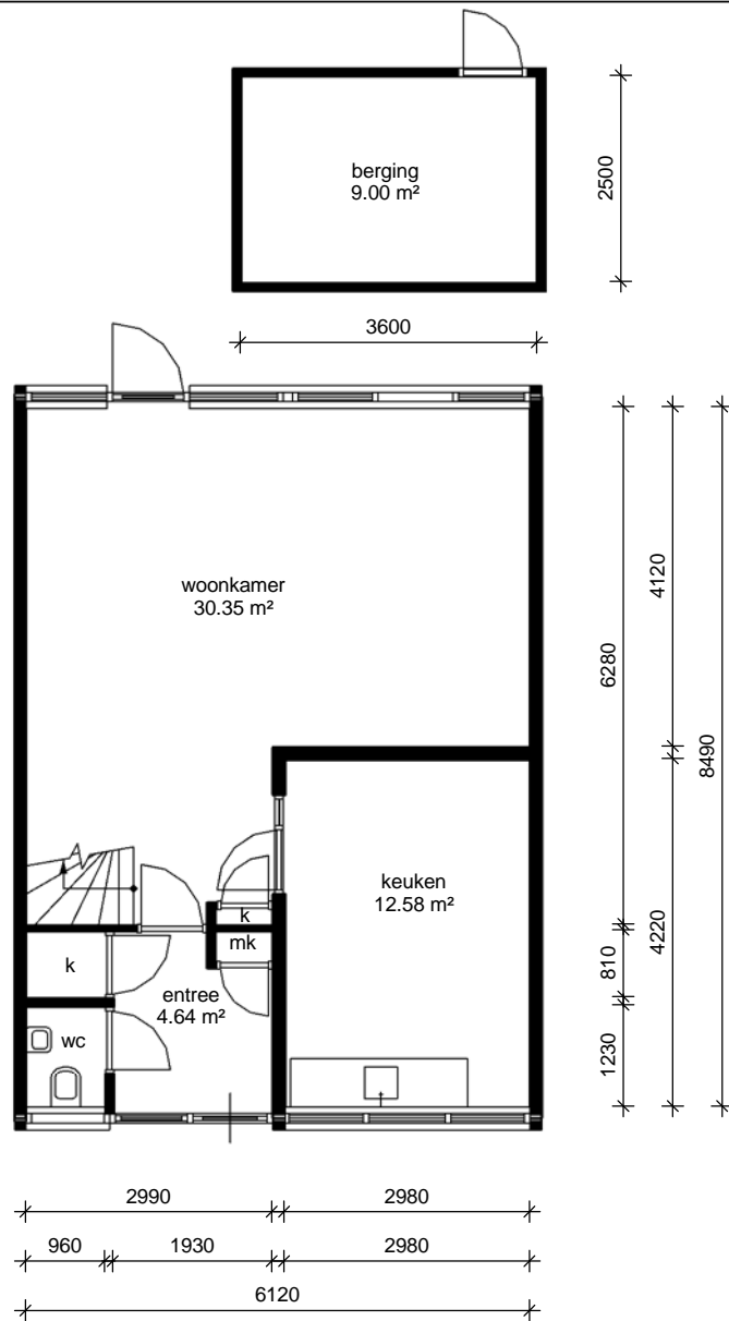
begane grond
