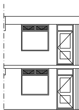
Voorgevel
