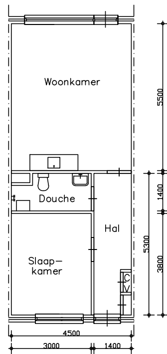
Begane grond
