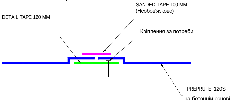
C-C ГОРИЗОНТАЛЬНИЙ НАХЛІСТ НА КІНЦІ РУЛОНУ Розріз
