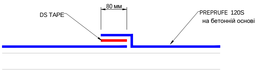
D-D АЛЬТЕРНАТИВНИЙ НАХЛІСТ НА КІНЦІ РУЛОНУ Розріз
