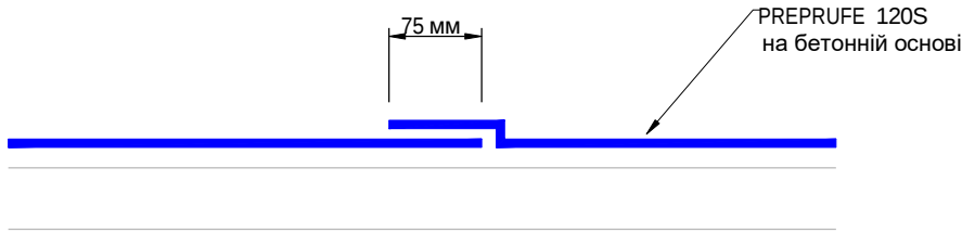
B-B ГОРИЗОНТАЛЬНИЙ НАХЛІСТ УЗДОВЖ КРОМКИ Розріз
