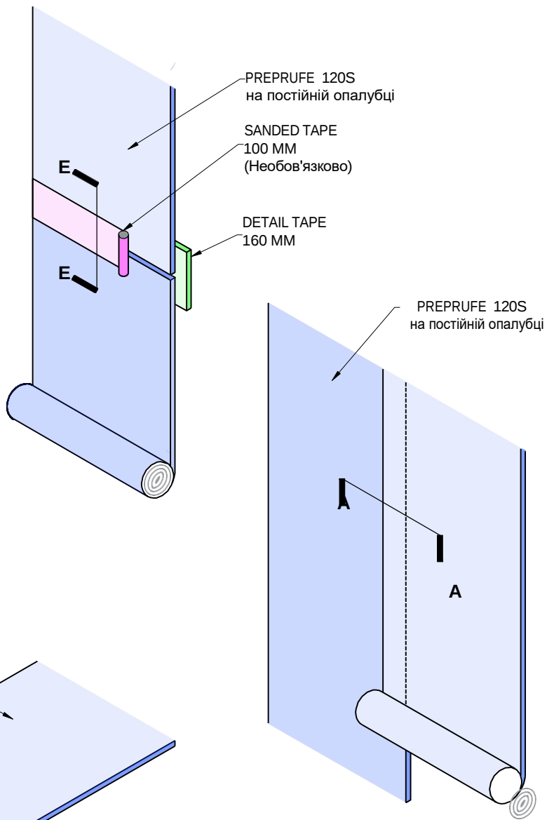
E-E ВЕРТИКАЛЬНИЙ НАХЛІСТ НА КІНЦІ РУЛОНУ Розріз
