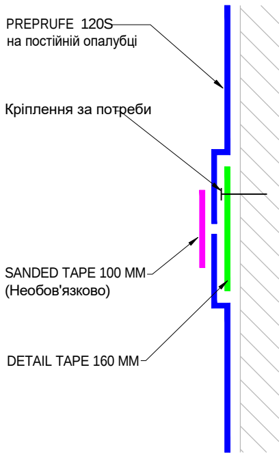
E-E ВЕРТИКАЛЬНИЙ НАХЛІСТ НА КІНЦІ РУЛОНУ Розріз
