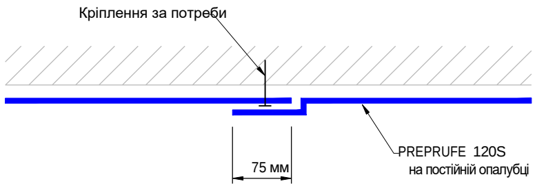
A-A ВЕРТИКАЛЬНИЙ НАХЛІСТ УЗДОВЖ КРОМКИ План / Розріз
