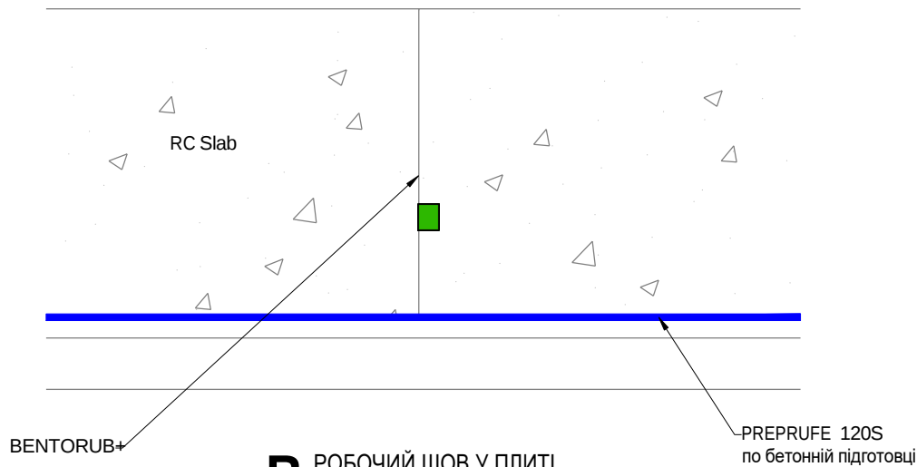
B РОБОЧИЙ ШОВ У ПЛИТІ Розріз
