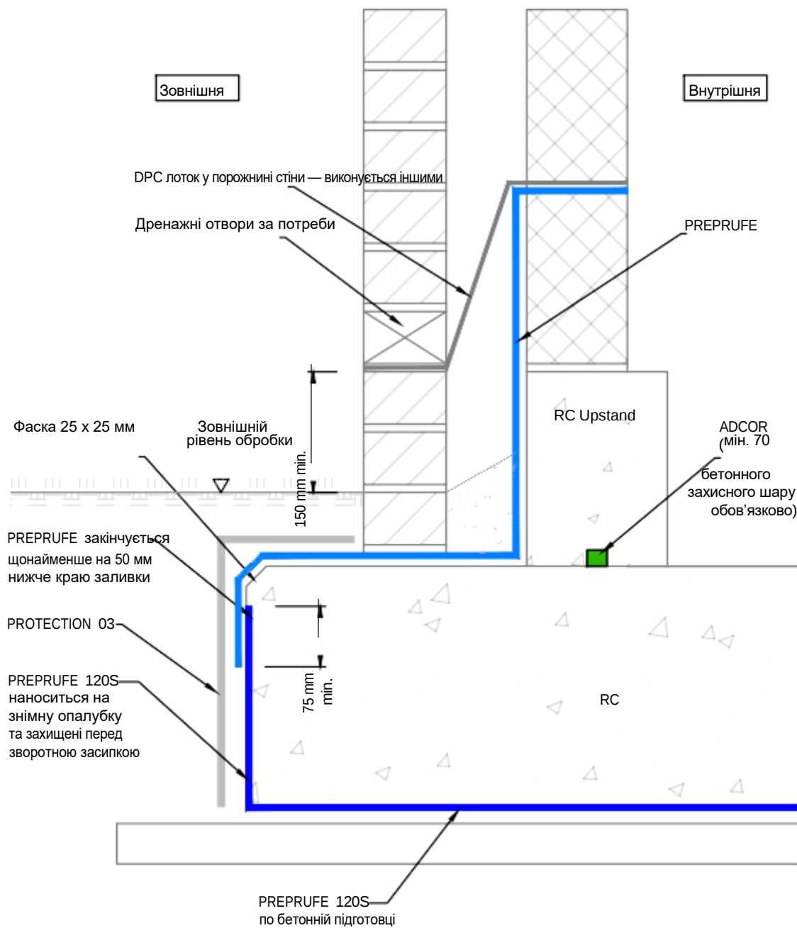
B ПРИМИКАННЯ ПО КРАЮ ПЛИТИ - PREPRUFE Розріз
