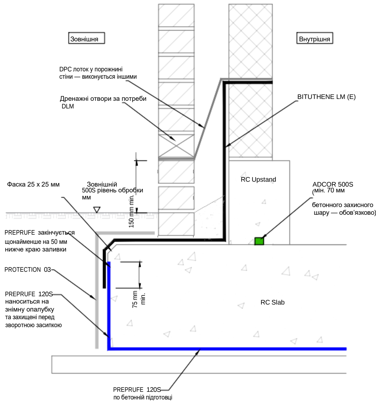
A ПРИМИКАННЯ ПО КРАЮ ПЛИТИ - BITUTHENE LM (E) DLM Розріз
