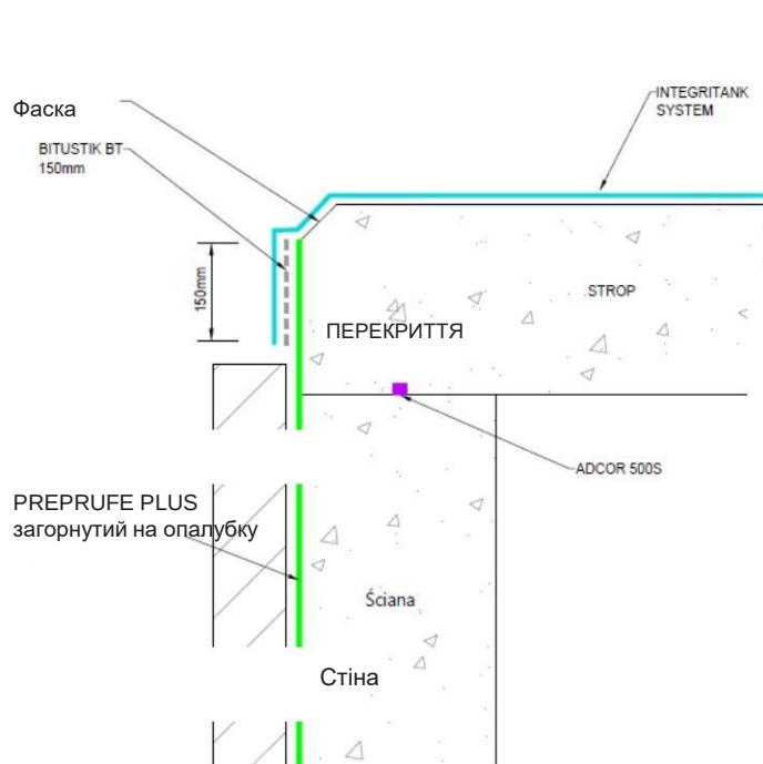
ДЕТАЛЬ З'ЄДНАННЯ СТІНИ ЗІ СТЕЛЕЮ SYSTEM PREPRUFE PLUS/INTEGRITANK — ПЕРЕРІЗ
