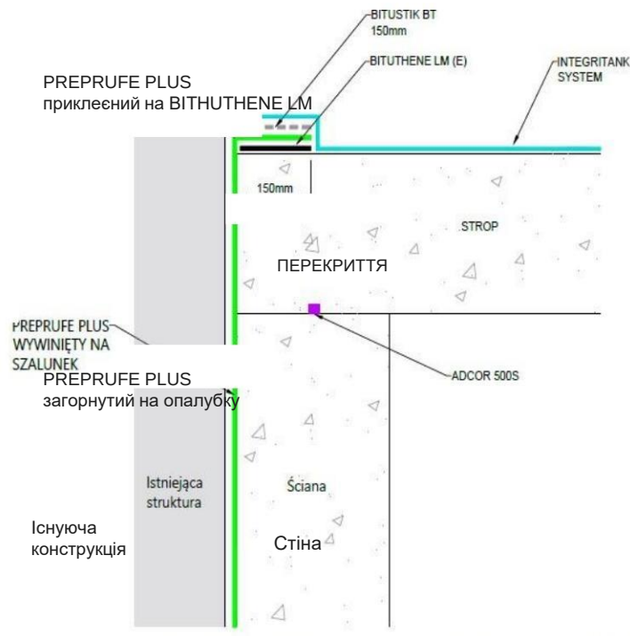
З'ЄДНАННЯ СТІНА-СТЕЛЯ SYSTEM PREPRUFE PLUS/INTEGRITANK ОПАЛУБКА НЕЗНІМНА/ОДНОСТОРОННЯ — ПЕРЕРІЗ
