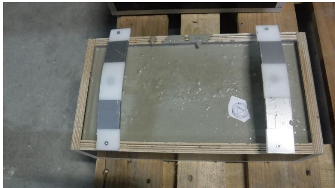
Фото 7 Зразок марковано ідентифікаційним знаком Kiwa BDA та готовий до твердіння у формі.
