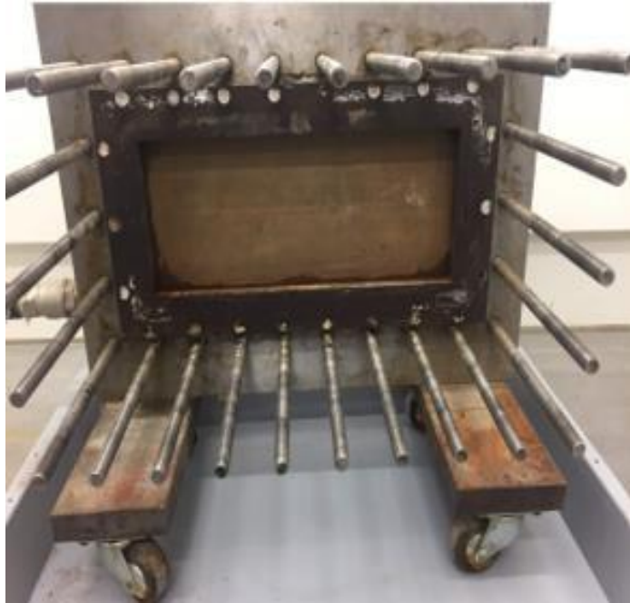
Фото 4 Випробувальне обладнання підготовлено для встановлення зразка.
