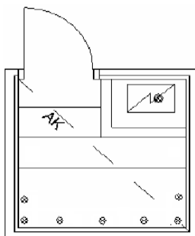
Periaatepiirustus
