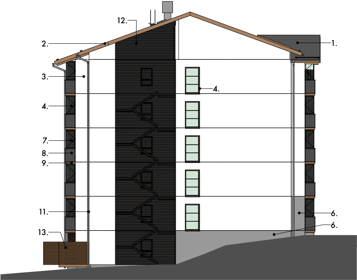
JULKISIVU POHJOISEEN
