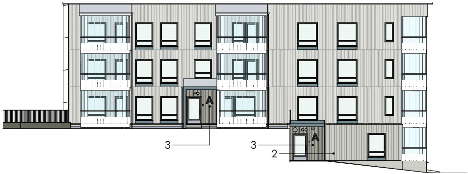
JULKISIVU KOILLISEEN
